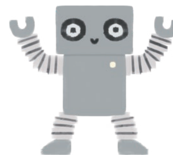
ロボット
